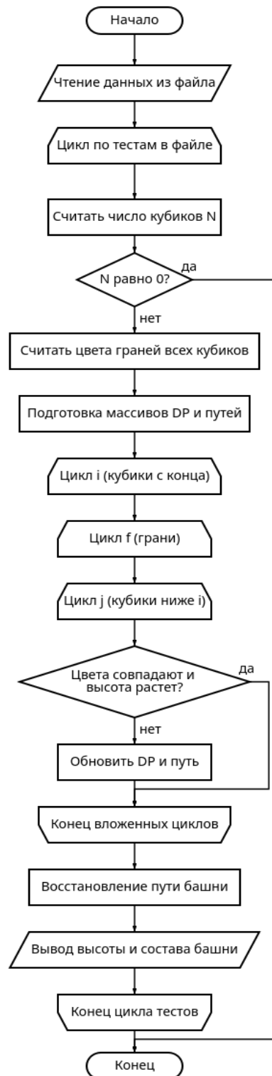
Рисунок 1 - Схема алгоритма.
