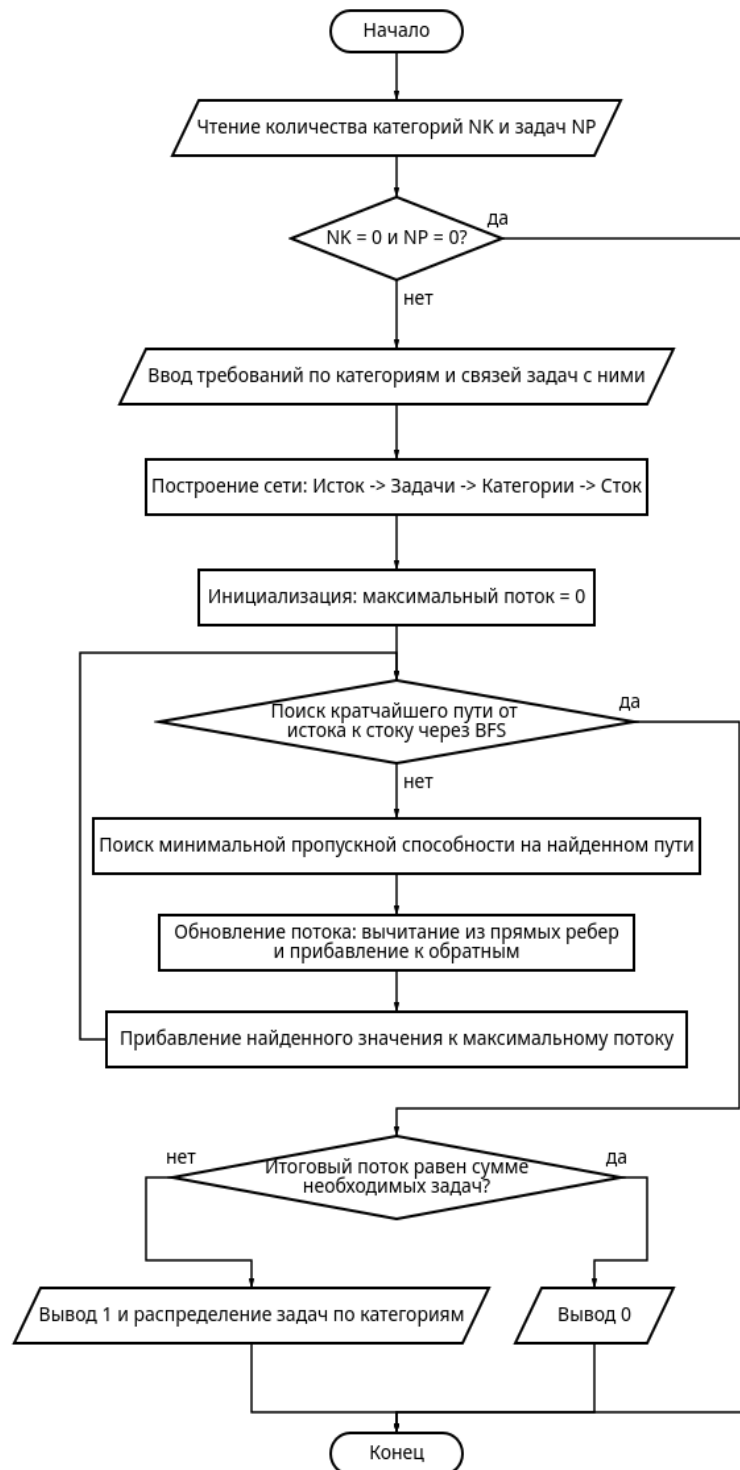
Рисунок 3 - Схема алгоритма.
